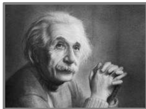
Albert Einstein
